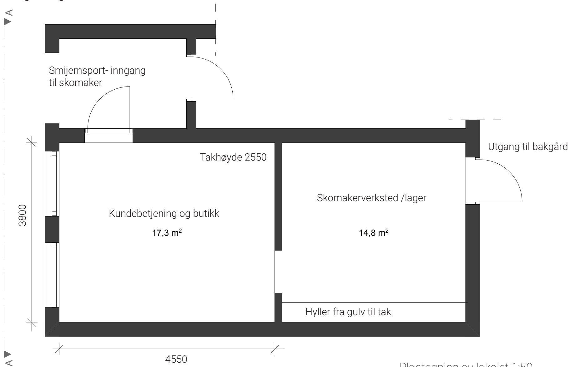
Plantegning av lokalet 1:50
